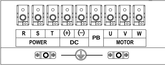
图 1-9 45~90kW 主回路端子示意图
