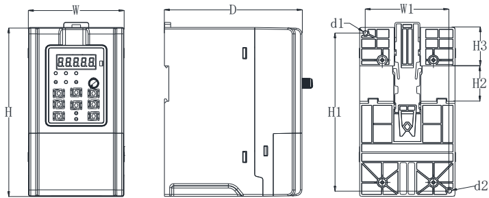
图 1-2 FR150A (0.2~22kW)产品尺寸示意图
