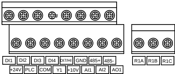
图 1-13 三相 380V (≥5.5kW)或单相 220V(≥4.0kW) 控制端子
