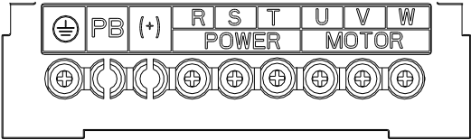
图 1-5 FR150A (0.7~4.0kW) 三相主回路端子
