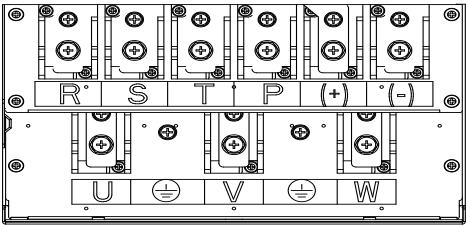
图 1-10 110~132kW 主回路端子示意图
