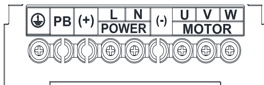
图 1-4 FR150A(0.2~2.2kW) 单相主回路端子
