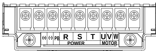
图 1-5 4.0kW 主回路端子示意图
