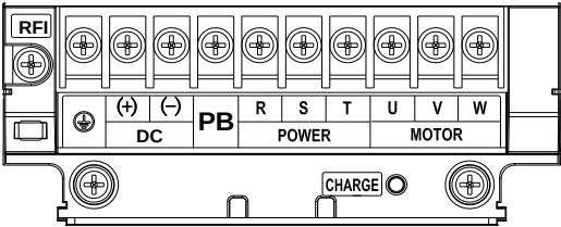
图 1-7 11~22kW 主回路端子示意图
