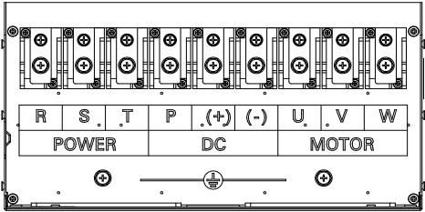
图 1-11 160kW 主回路端子示意图
