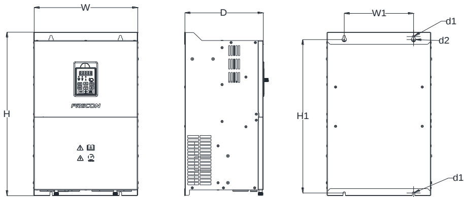
图 1-3 FR150A (30~160kW)产品尺寸示意图
