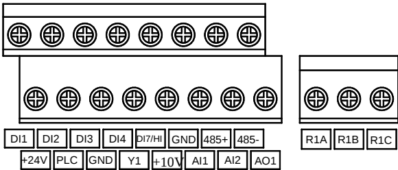
图 1-12 三相 380V (<5.5kW)或单相 220V(<4.0kW) 控制端子示意图
