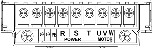
图 1-6 5.5~7.5kW 主回路端子示意图
