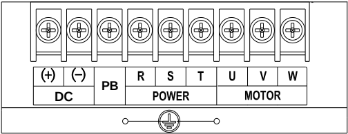
图 1-8 30~37kW 主回路端子示意图
