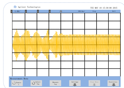
振荡抑制波形图
