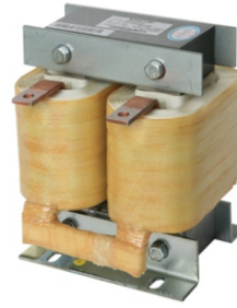
直流电抗器
