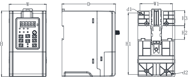
□ FR150A (0.2~22kW) 安装尺寸
