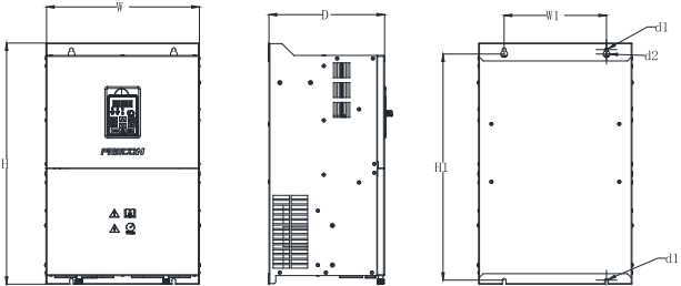
□ FR150A (30~160kW) 安装尺寸
