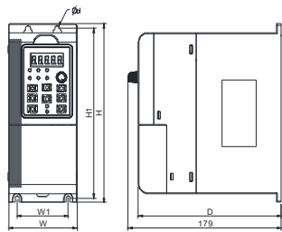
0.7-2.2Kw结构示意图
