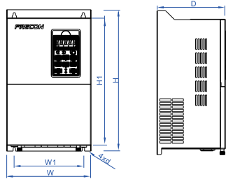
30-560Kw结构示意图
