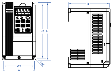
4-22Kw结构示意图
