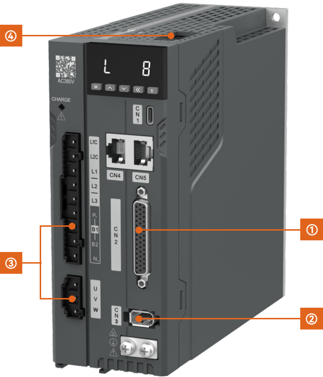
①CN2控制端子定义
