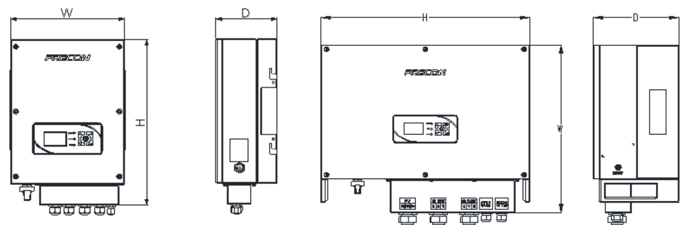
图1-4 产品尺寸示意图 (≤22KW)
