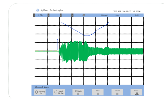
转速追踪输出频率和电流波形图
