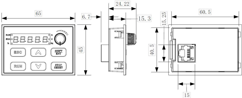
图 2-3 操作键盘尺寸图
