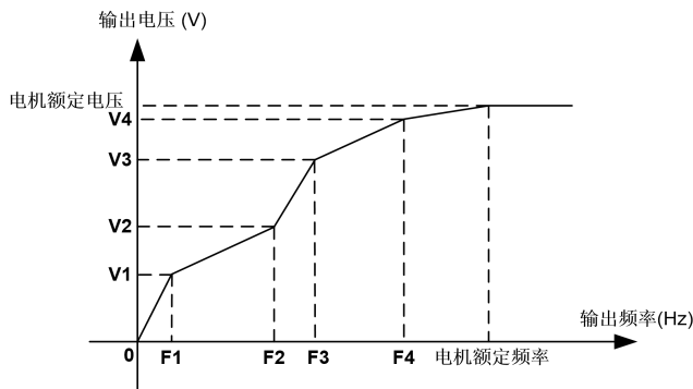
图 6-26 多点 VF 曲线示意图
