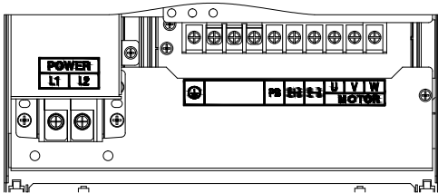
4.0-11kW 主回路端子
