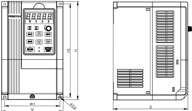
图 1-3 0.7～22kW 壁挂安装示意图
