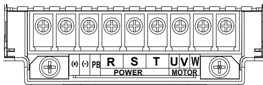
图 1-7 0.75~5.5kW 主回路端子示意图
