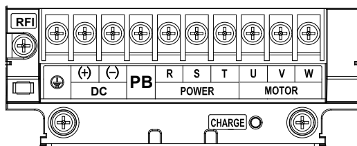
图 1-8 7.5~22kW 主回路端子示意图
