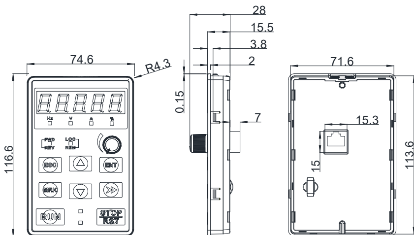
图 c-2 7.5~450kW 操作键盘尺寸图
