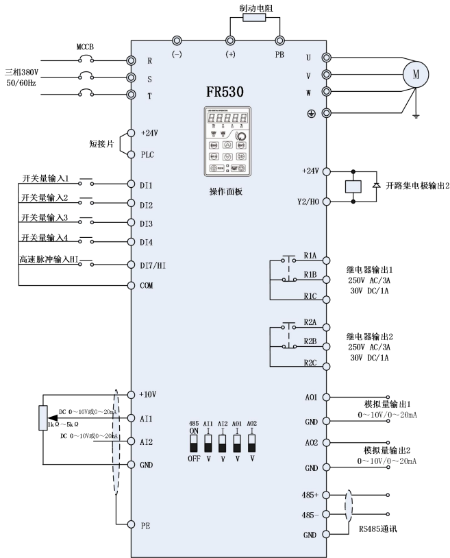
图 1-6 FR530 变频器接线示意图
