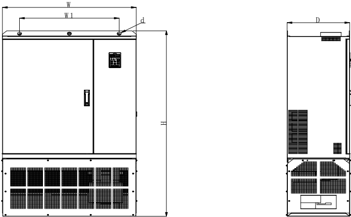
图 1-7 450～560kW 壁挂安装示意图
