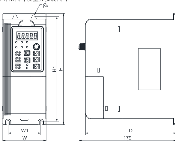
图 1-3 0.7~2.2kW 壁挂安装示意图
