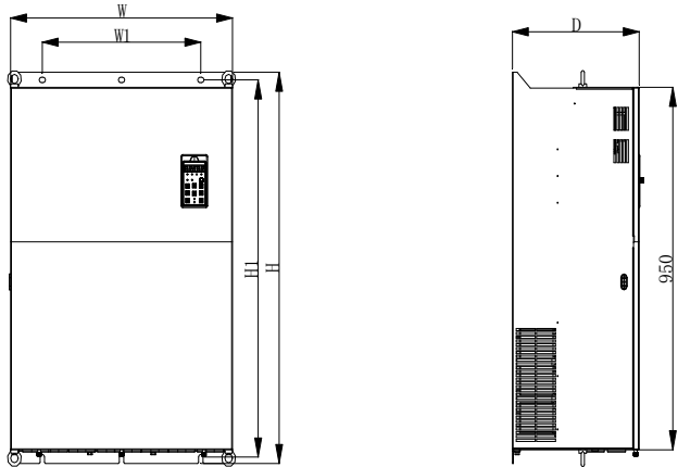
图 1-6 315~400kW 壁挂安装示意图
