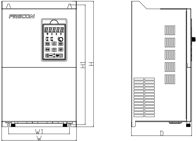
图 1-5 30~280kW 壁挂安装示意图
