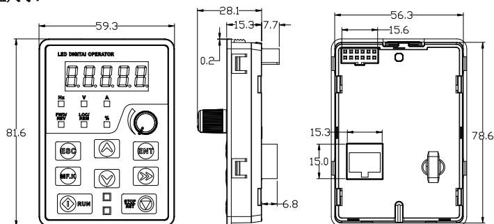
图 c-1 0.7~5.5kW 操作键盘尺寸图
