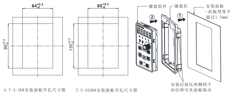
图 c-3 4~450kW 键盘外置安装开孔尺寸图
